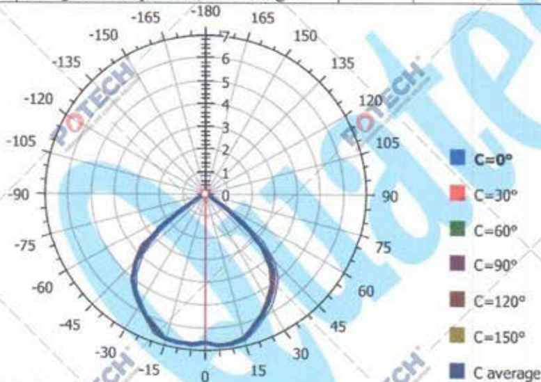
Hình 1: Đồ thị phân bố cường độ sáng (Calculated Luminous Intensity / kcd)
